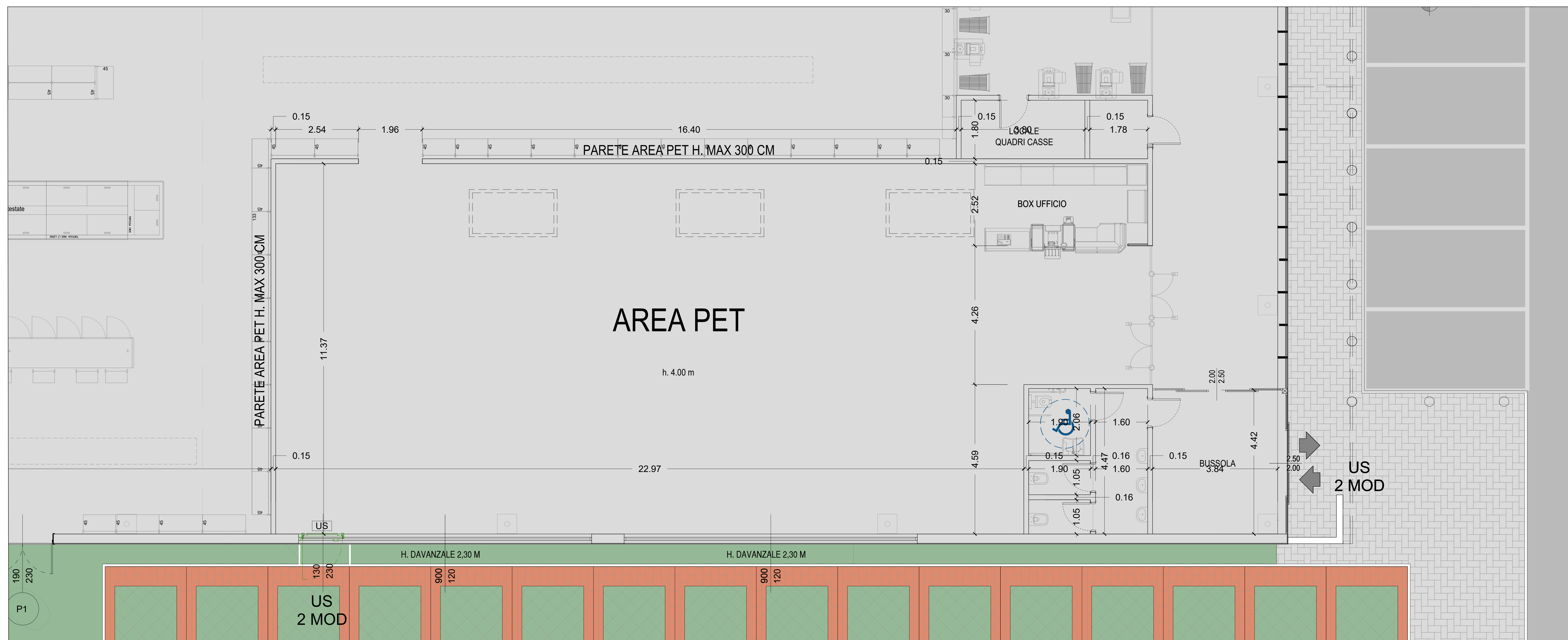
PARTICOLARE B
