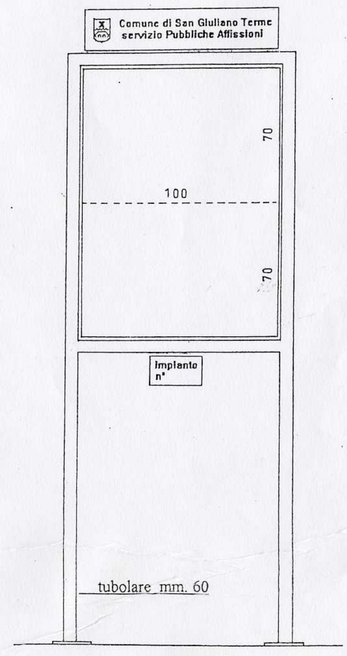
"standardo tipo B"
