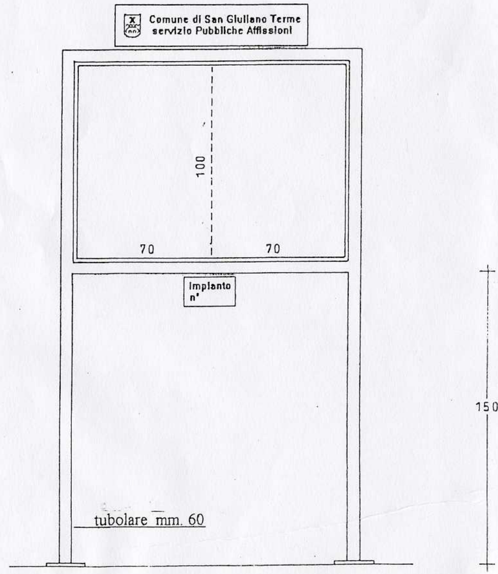
"standardo tipo A"
