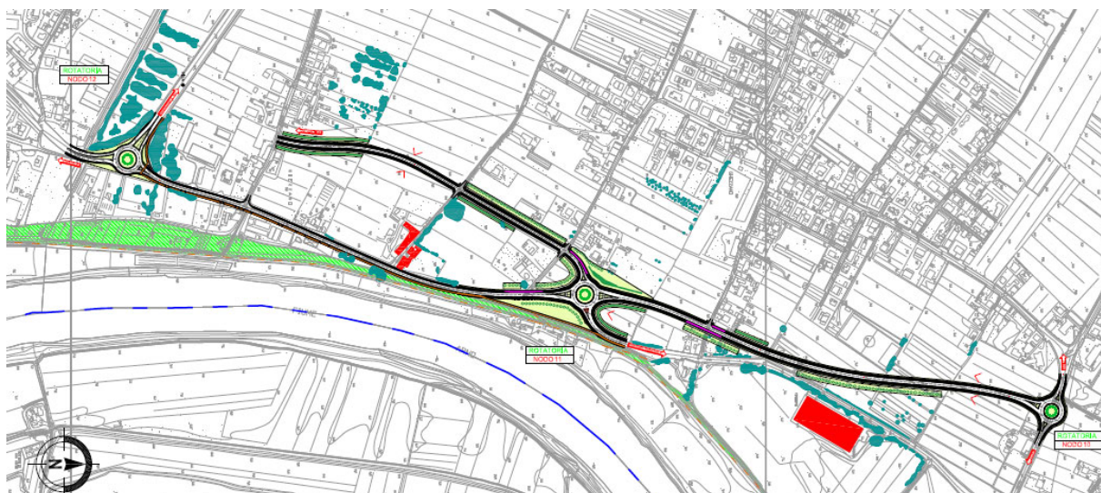
Figura 28 – nodi 10-12 e beni tutelati (in rosso)
