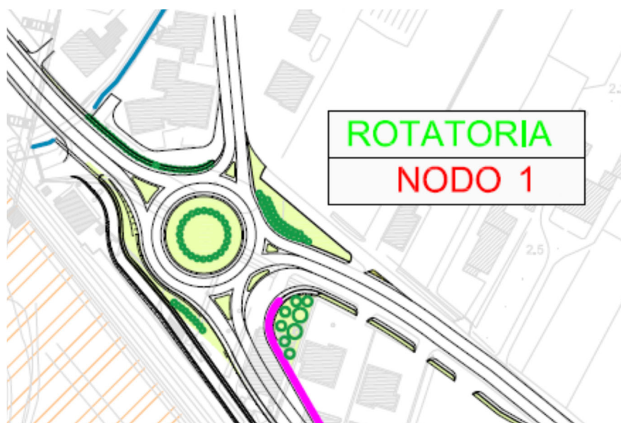
Figura 44 – Nodo 1, dettaglio delle mitigazioni in planimetria
