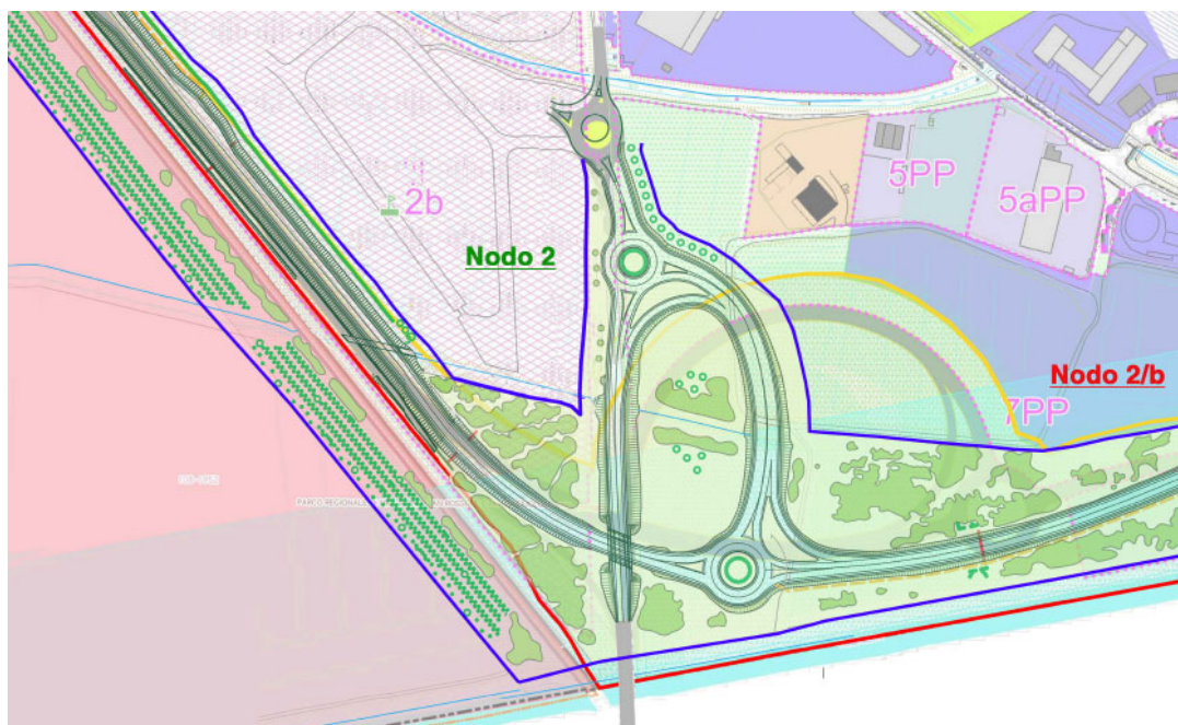
Figura 77 – Sovrapposizione tracciato Progetto Definitivo (in verde) e tavola del Piano Operativo Comunale di San Giuliano Terme nel Nodo 2 (Lotto 1-3)
