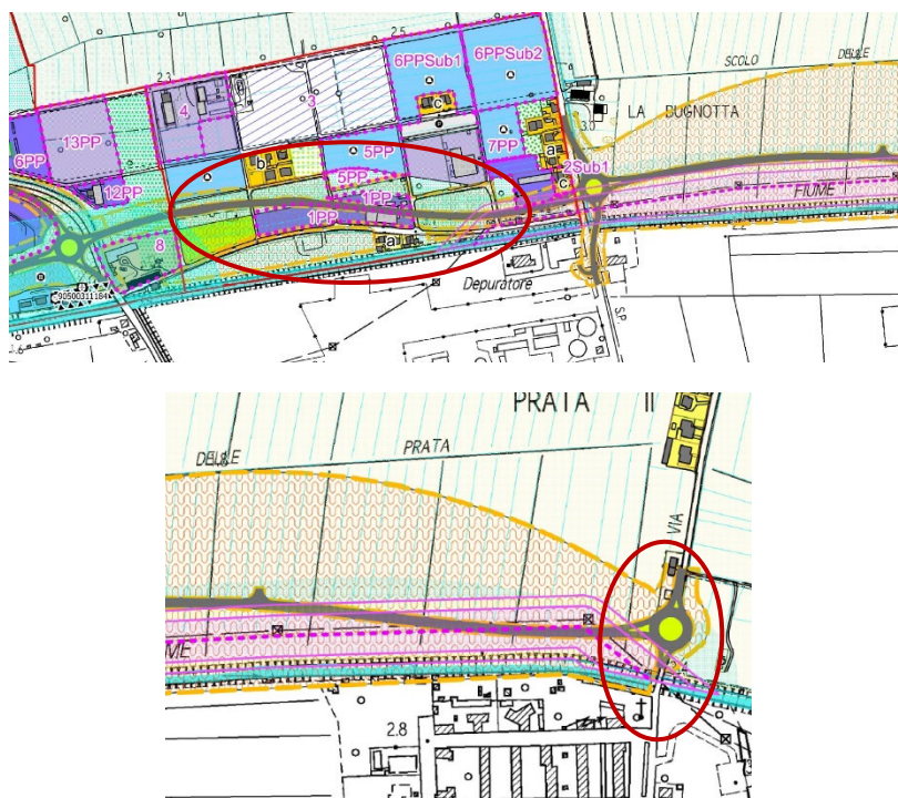
Figura 42 – Estratto di cartografia per la Variante: Progetto Definitivo Lotto funzionale 3-5 (nodi 3, 4 e 5) e POC
