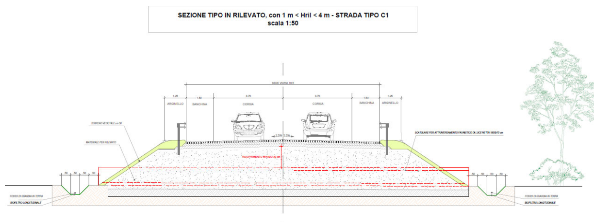
Figura 48 – Sezione tipo nel tratto tra i nodi 1 e 2 – Progetto Definitivo: eliminazione del terrapieno “tipo dune”
