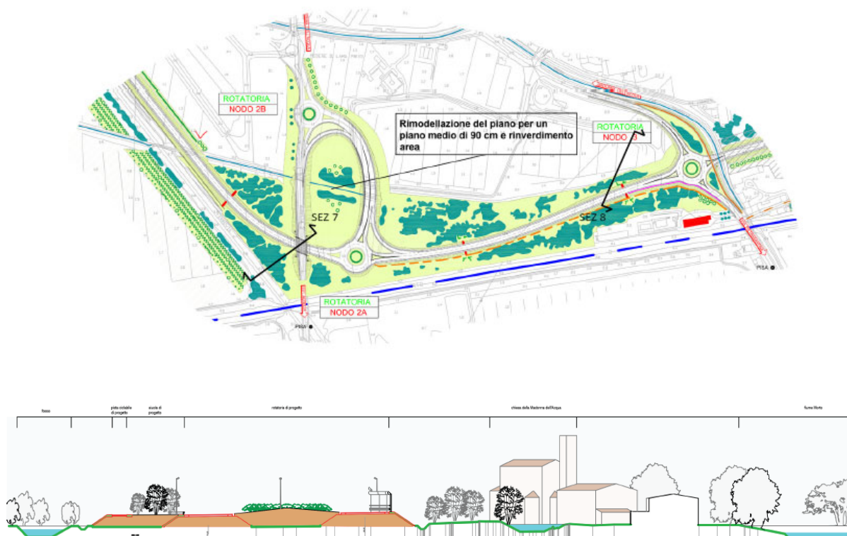
Figura 7 – Sezione sul tratto 2-3 (sezione 8)
