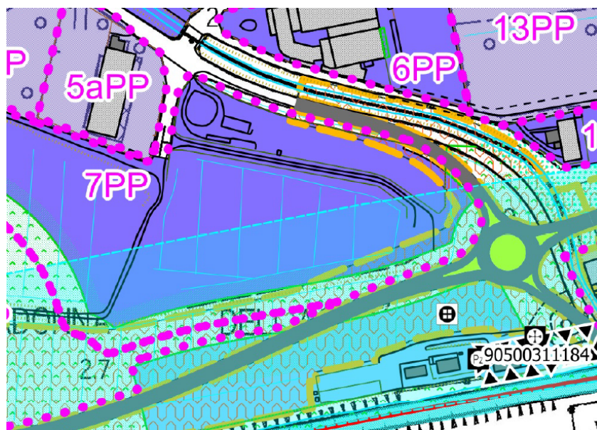
Figura 78 – Estratto di tavola per la Variante urbanistica – sovrapposizione tracciato Progetto Definitivo e tavola del Piano Operativo Comunale di San Giuliano Terme nel Nodo 3 (Lotto 1-3, 3-5)
