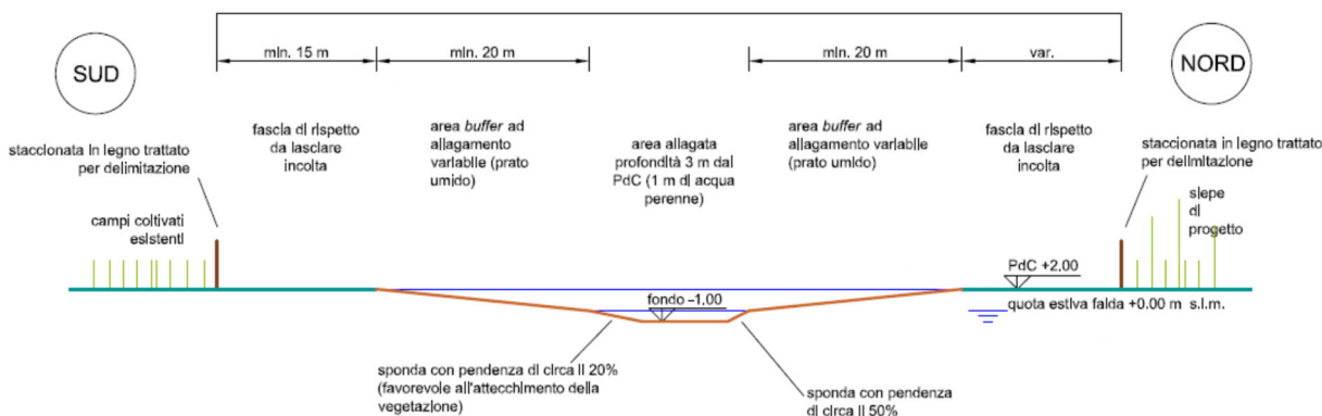
Figura 46 – Sezione area umida di progetto
