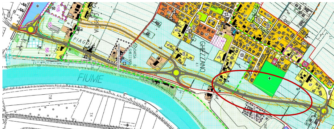
Figura 43 – Estratto di cartografia per la Variante: Progetto Definitivo Lotto funzionale 10-12 (nodi 10, 11 e 12) e POC
