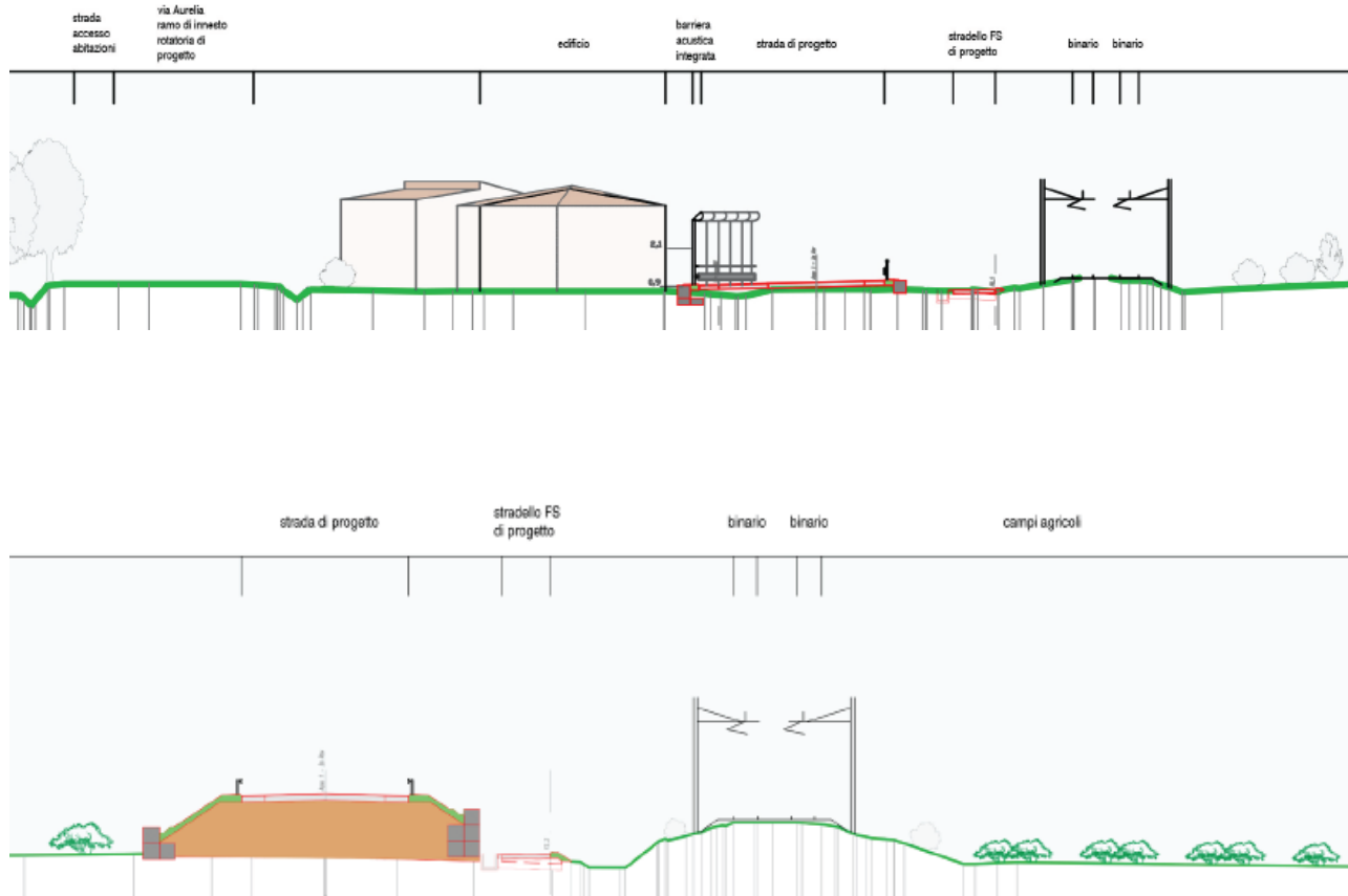
Figura 5 – Sezioni sul tratto 1-2 (sezioni 3 e 6)
