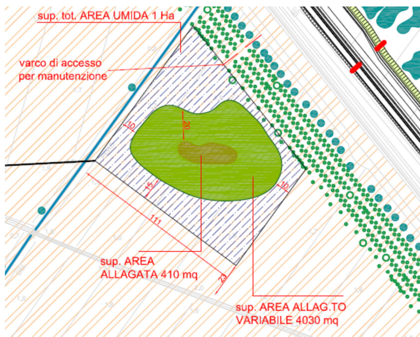
Figura 45 – Planimetria area umida di progetto
