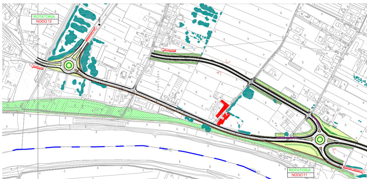
Figura 54 – Planimetria nodi 11-12 (in rosso elementi di pregio storico-culturale)
