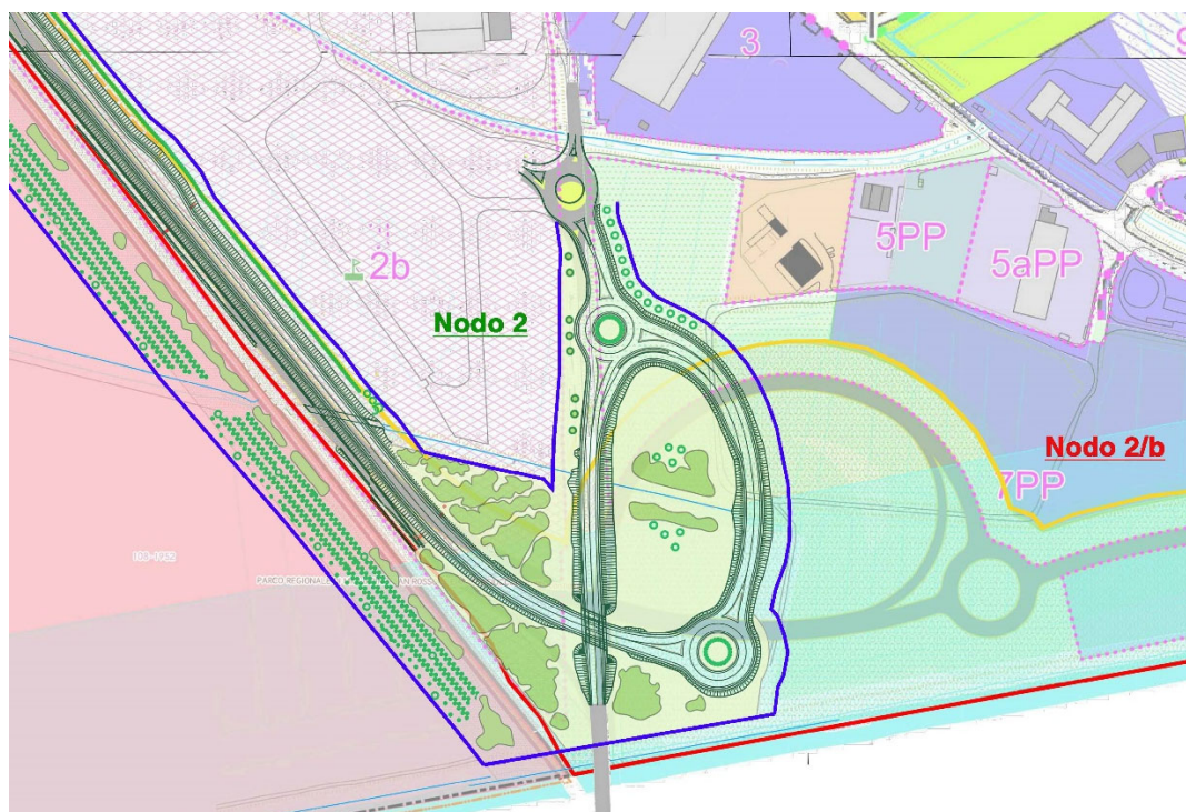
Figura 76 – Sovrapposizione tracciato Progetto Definitivo (in verde) e tavola del Piano Operativo Comunale di San Giuliano Terme nel Nodo 2 (Lotto stralcio 1-2)
