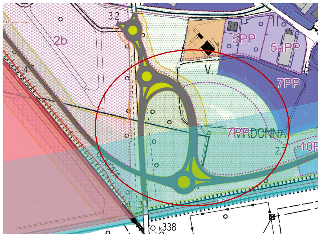
Figura 40 – Estratto di cartografia per la Variante: Progetto Definitivo Lotto stralcio 1-2 (nodo 2) e POC
