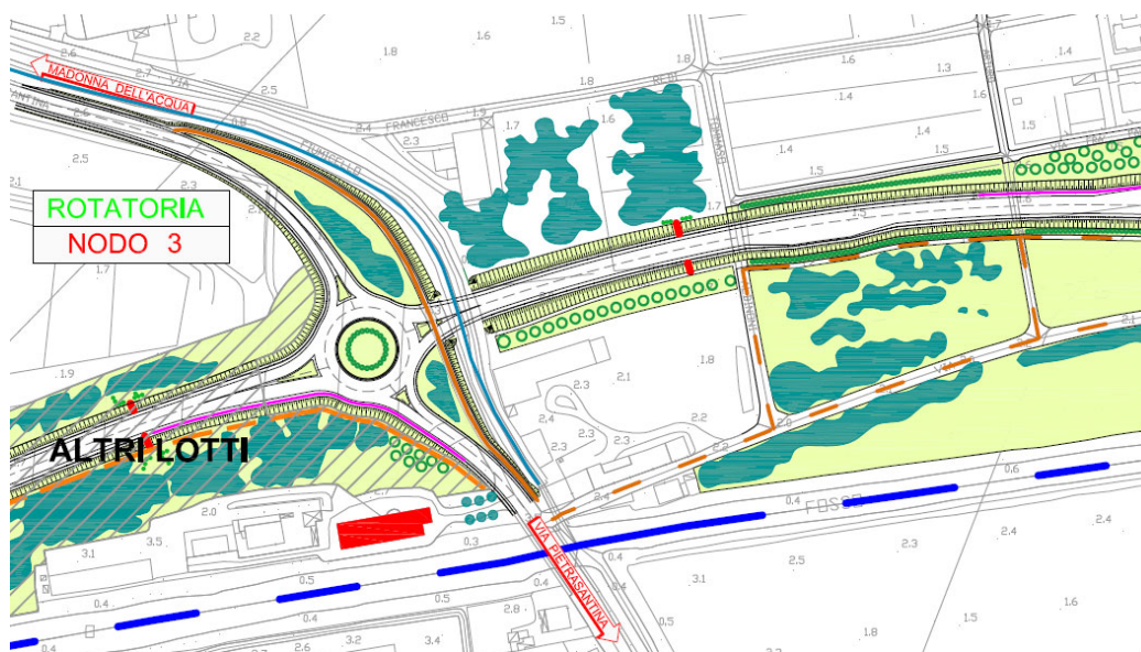
Figura 51 – Planimetria in corrispondenza del nodo 3
