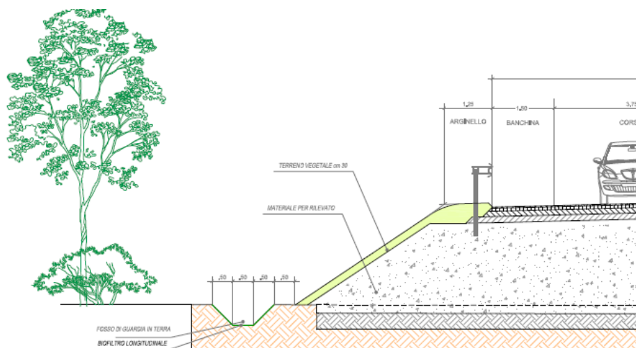
Figura 56 – Sezione tipo in presenza di biofiltro longitudinale
